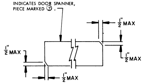
BEVEL - CUT
