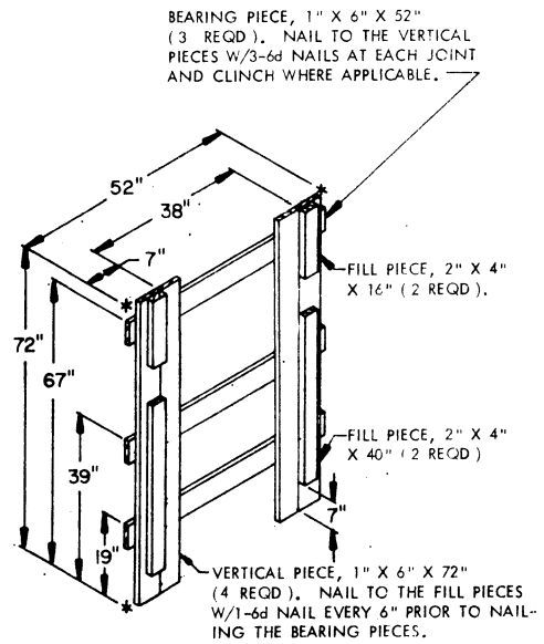
CENTER FILL GATE
