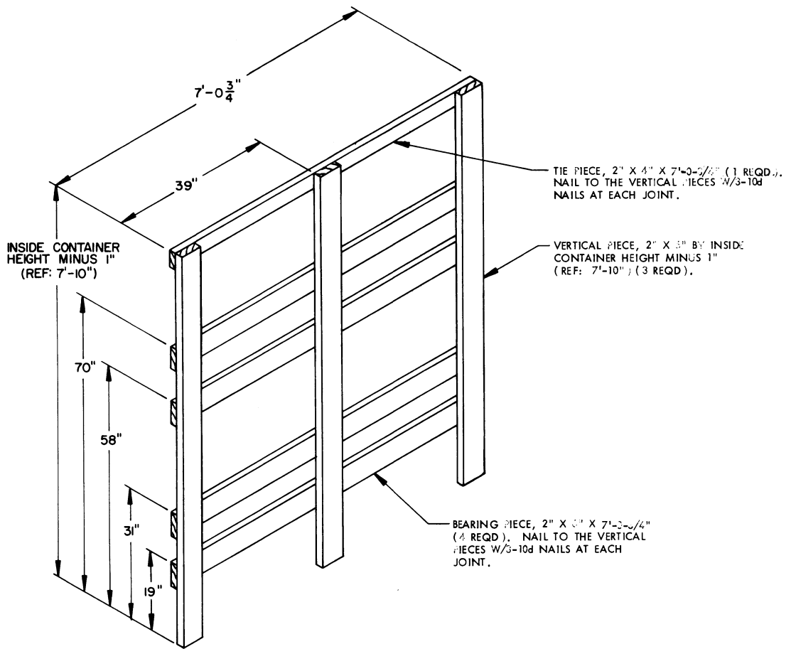
SIDE FILL ASSEMBLY
