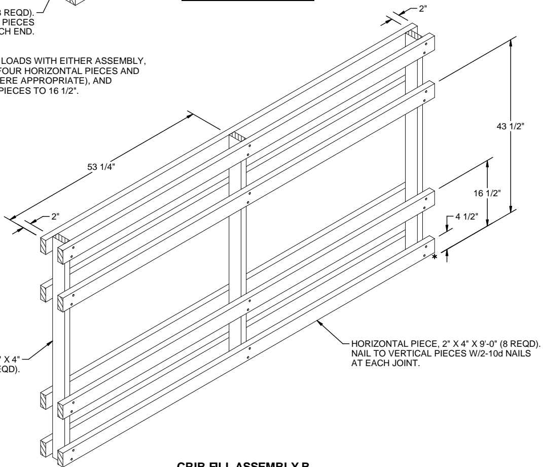
CRIB FILL ASSEMBLY B
