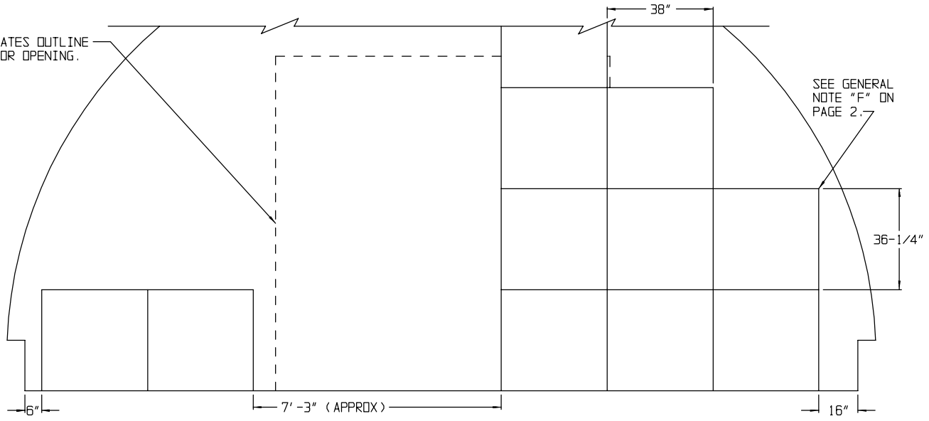
SECTION 0-0
