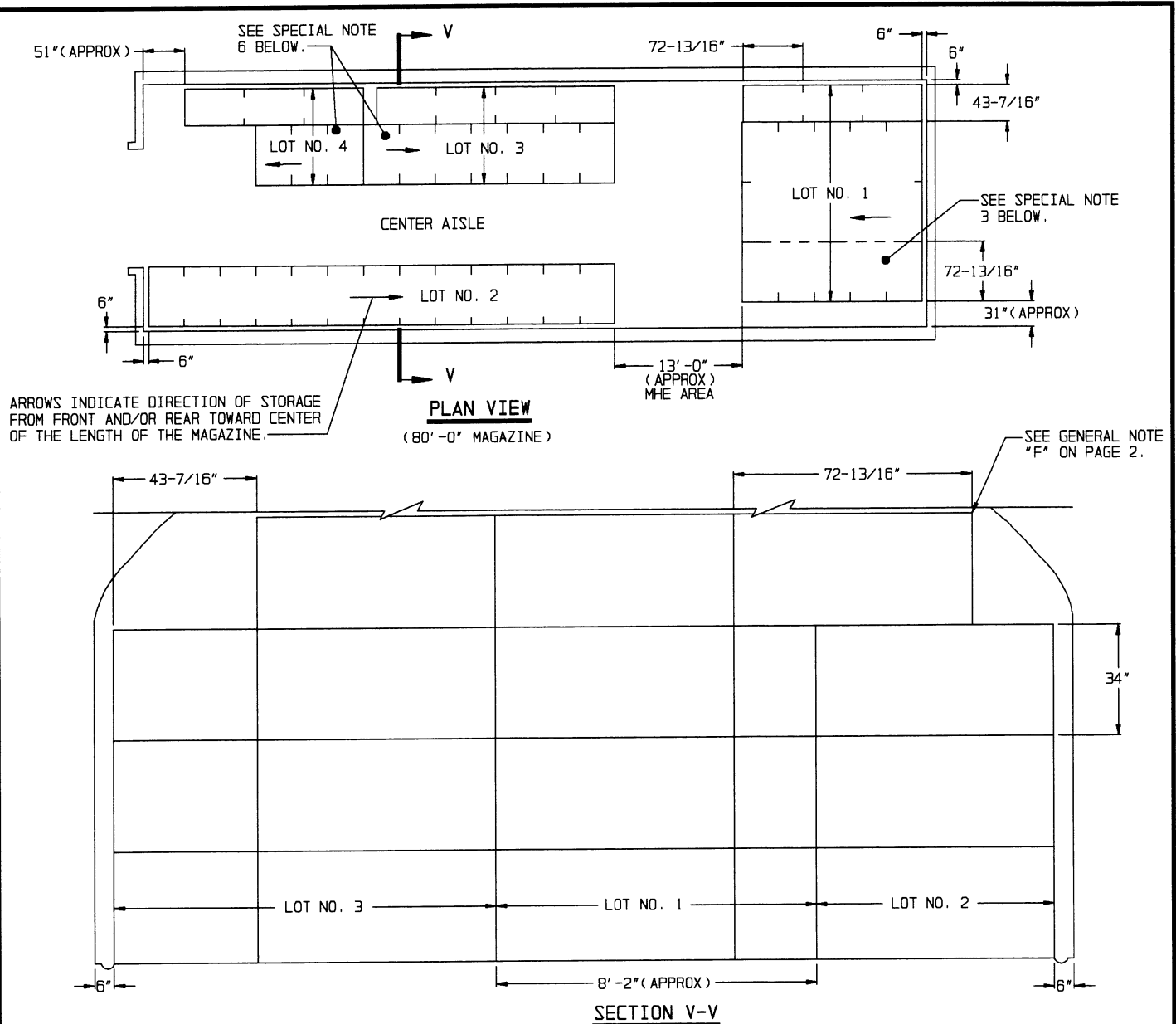
SECTION V-V
