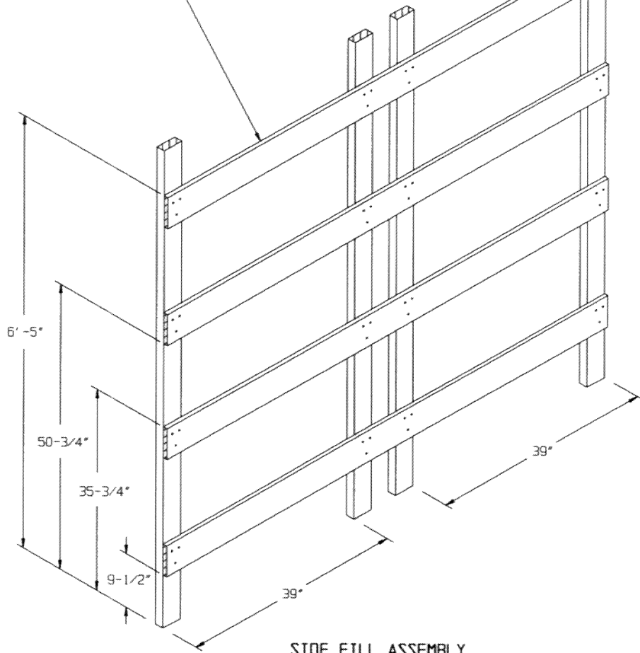
SIDE FILL ASSEMBLY
