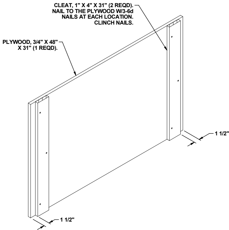
SEPARATOR GATE
