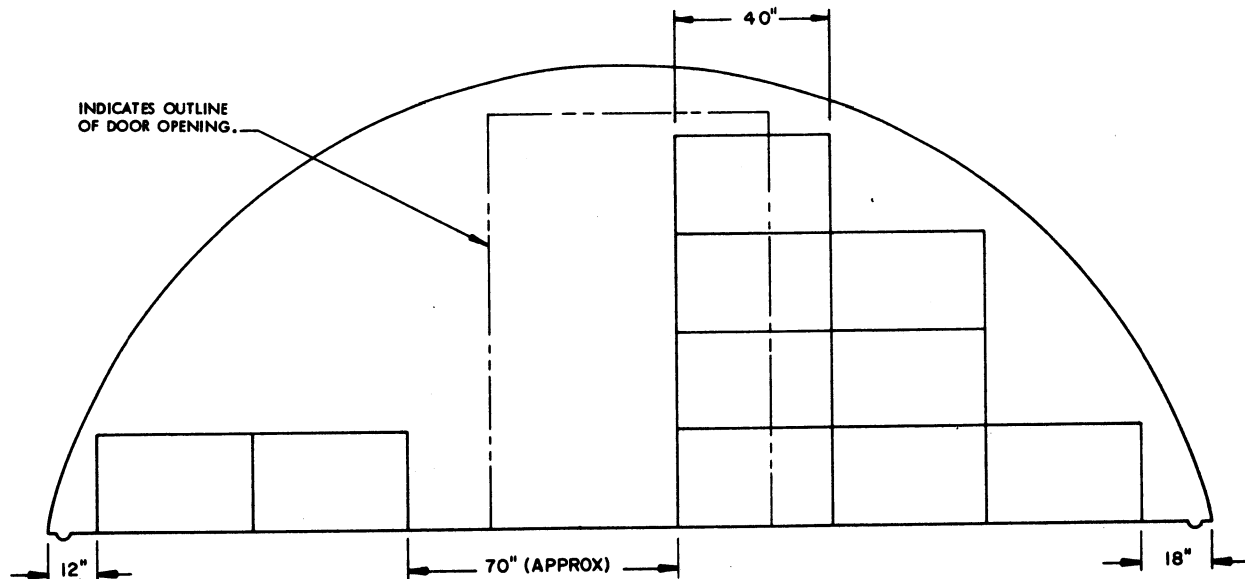
SECTION D-D
