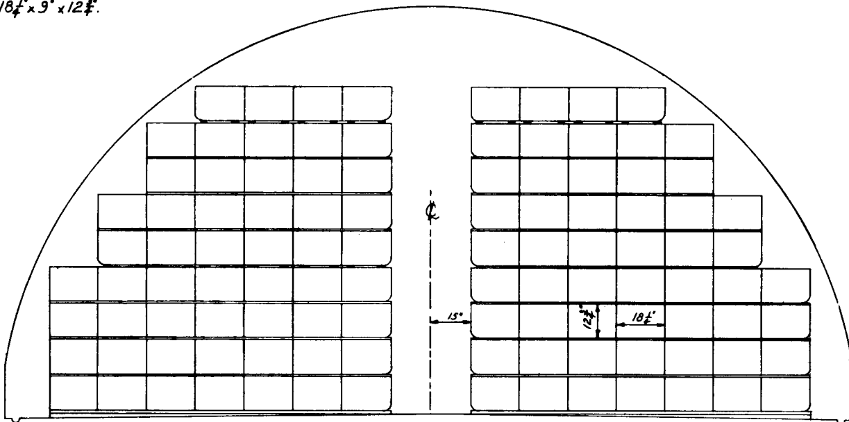
ELEVATION - STACK 'B'
